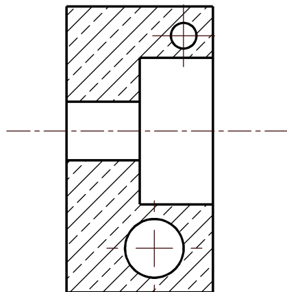
COUPE A-A
